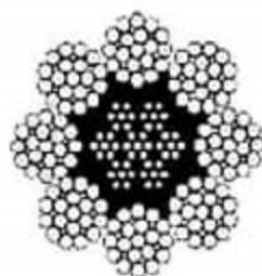
8xFi(25)IWRC
