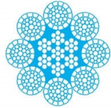
8 x P.WS{36:1+7+(7+7)+14} + IWRC
