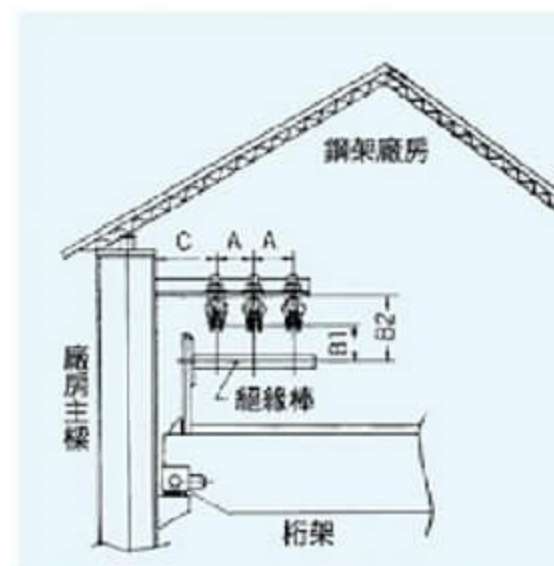
• 立式高架施工法 (Above)
