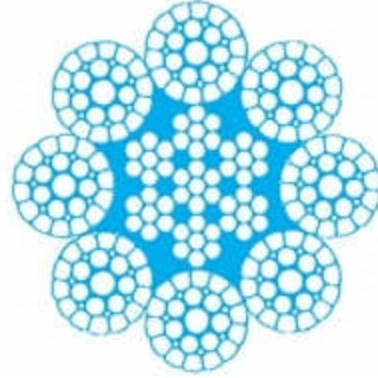
8 x P.Fi{29:1+7+(7)+14} + IWRC
