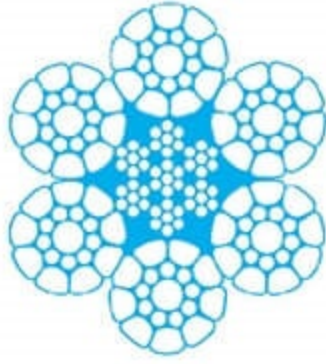
6 x P.S{19:1+9+9} + IWRC
