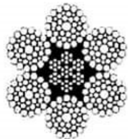
6xWS(41)IWRC
