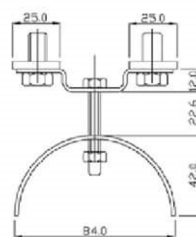
KY-BC4200 C40末端夾線器 End Cable Clip KY-BCS4200白鐵
