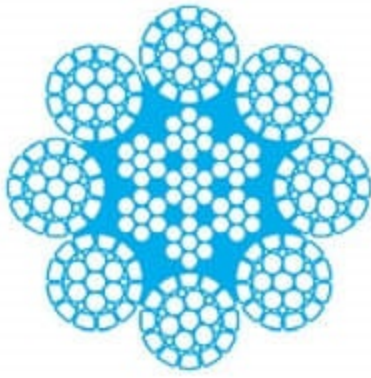
8 x P.Fi{25:1+6+(6)+12} + IWRC
