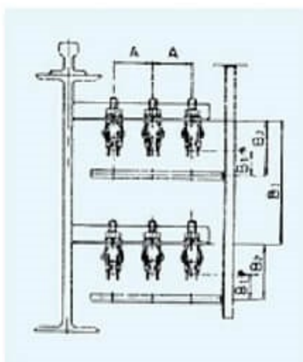
• 立式雙層施工法 Vertical (Double)
