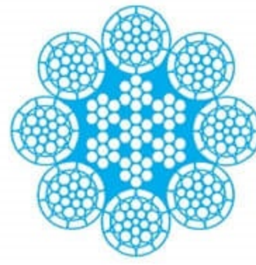
8 x P.WS{26:1+5+(5+5)+10} + IWRC
