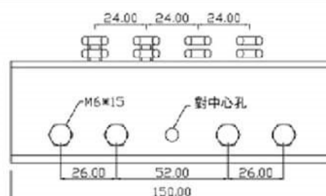
KY-BC4300 C40接頭 Track Coupler KY-BCS4300白鐵
