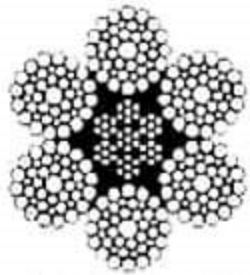
6xWS(41)IWRC
