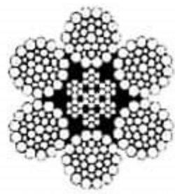
6xWS(36)IWRC
