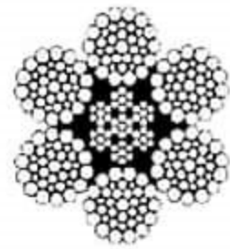
6xWS(36)IWRC
