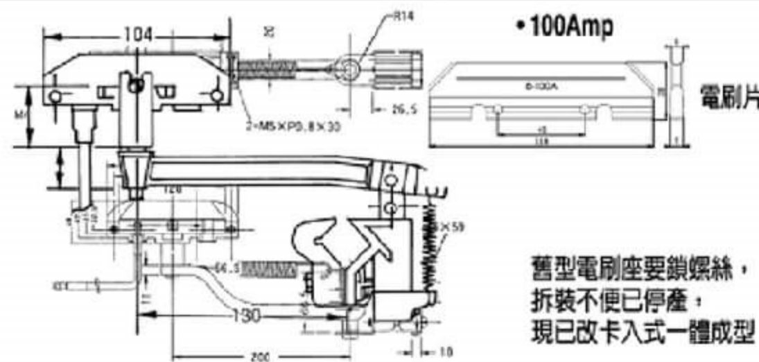
•100Amp •40Amp 電刷片 舊型電刷已停產 KY-AXE0804 KY-AXE0810 8字集電架40Amp 100Amp 鋁單臂集電架
