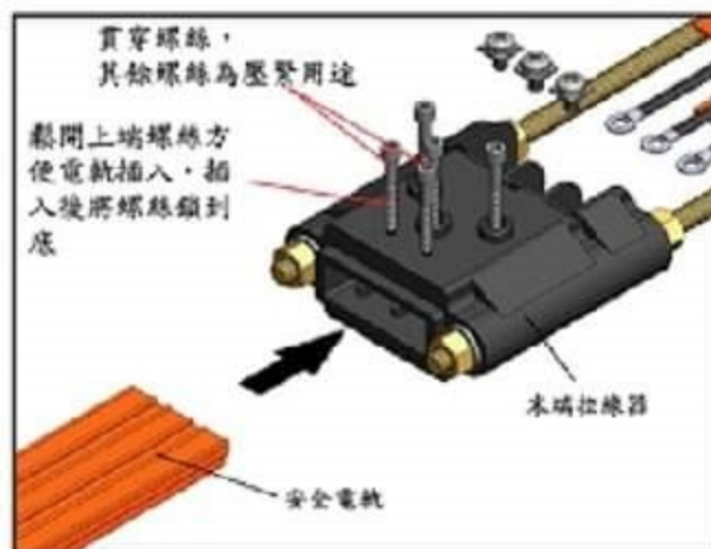
4-1 以 3P 電軌作為安裝範例
