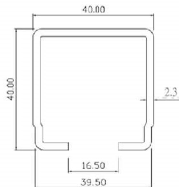
KY-BC4030 C40型軌道 C Track KY-BCS4030白鐵
