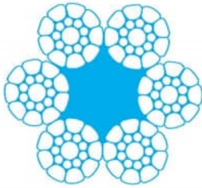
6 x P.S{19:1+9+9} + FC
