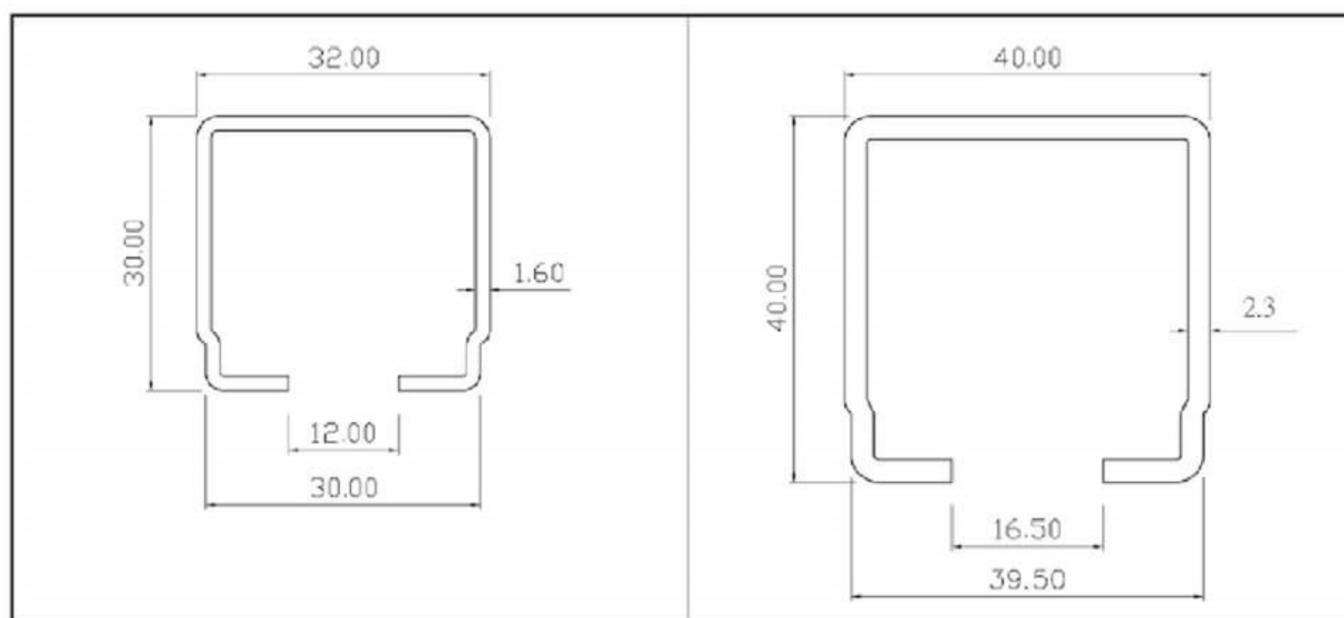
C30軌道斷面圖
