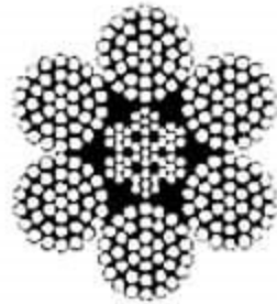
6x37IWRC
