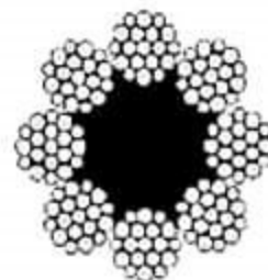
8xW(19)FC
