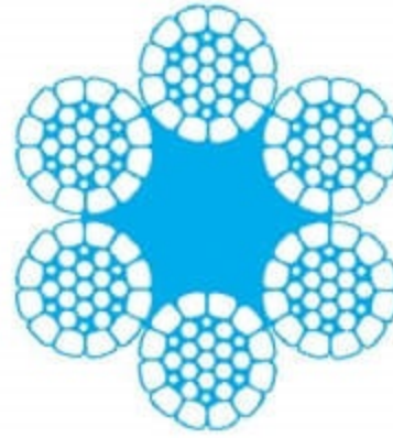
6 x P.WS{31:1+6+(6+6)+12} + FC
