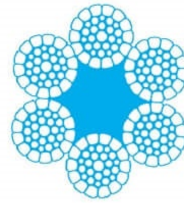
6 x P.WS{36:1+7+(7+7)+14} + FC
